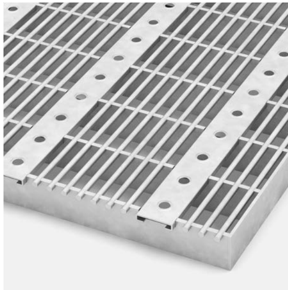
AR1-25 med skrabeliste af stansede stålprofiler.
