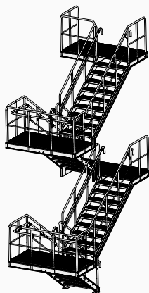
Flerløbstrappe
